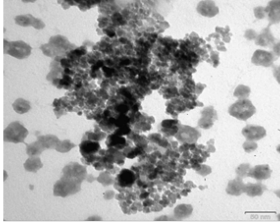
Şekil 3: AgNP'lerin TEM Görüntüleri
