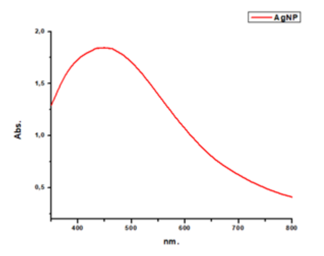
Şekil 1: AgNP'lerin UV-Vis Absorpsiyon Spektrumları
