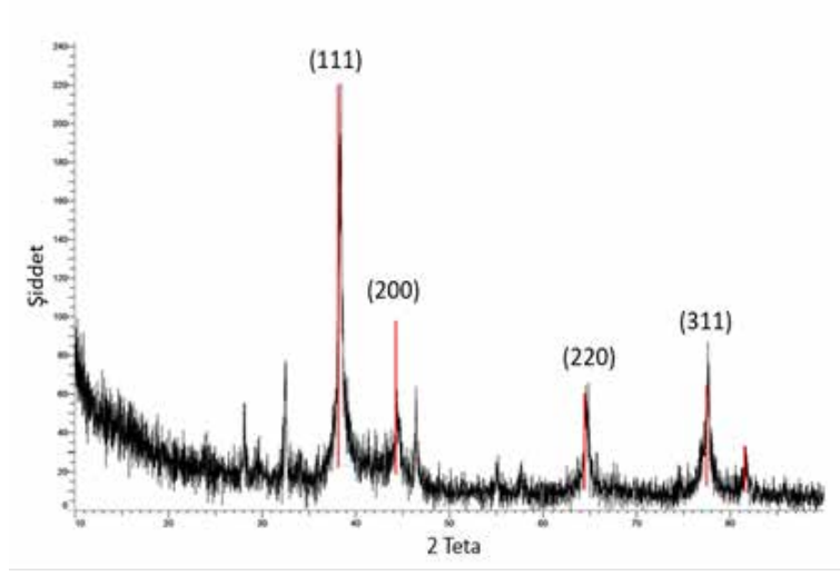
Şekil 2: AgNP’lerin XRD Görüntüleri
