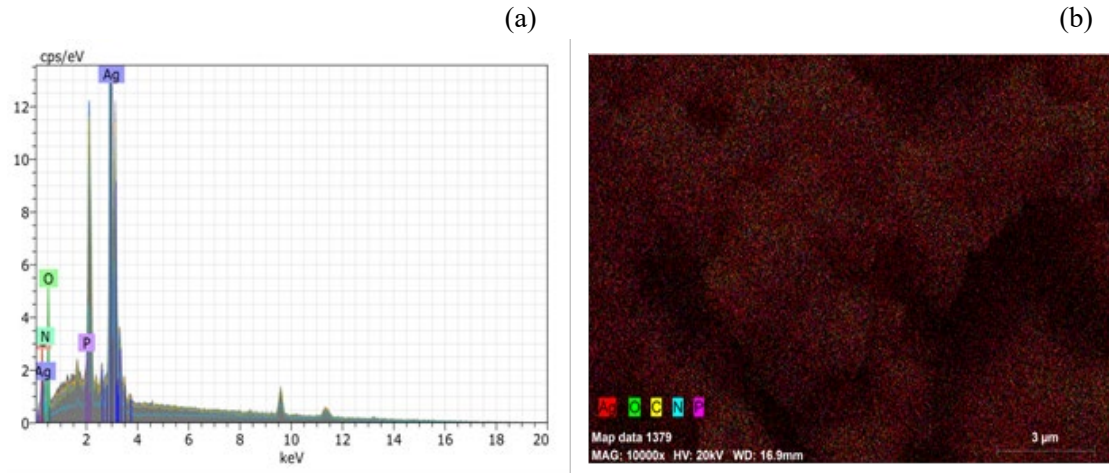
Şekil 4: a) AgNP'lerin EDX Analizi b) Elementel Dağılım c) Elementel Haritalama
